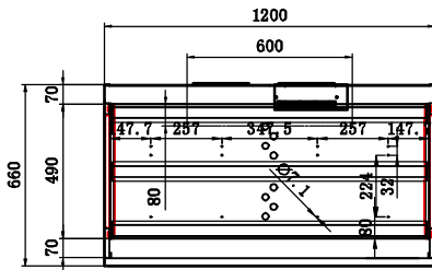
Draufsicht
