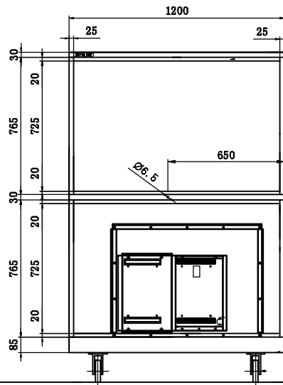
Rückansicht
