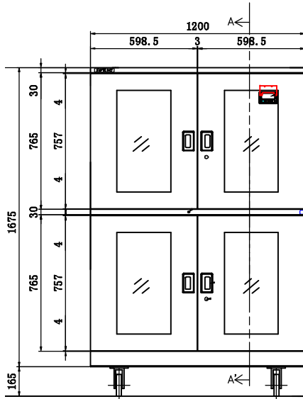
Frontansicht
